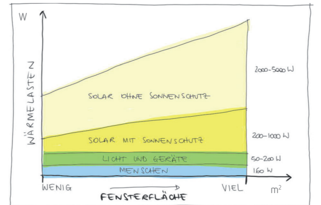
Abb. 2. Wärmeeintrag in einem Raum im Sommer
