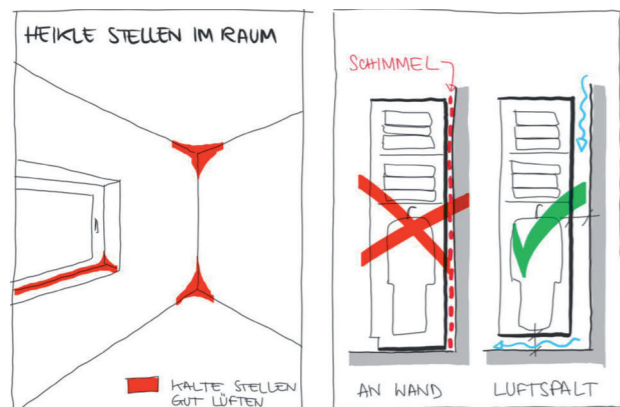
Abb. 4. Risikozonen für Schimmelpilzbildung
