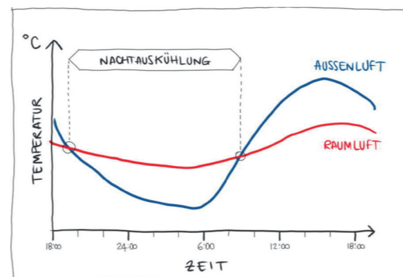
Abb. 7. Temperatureinfluss
