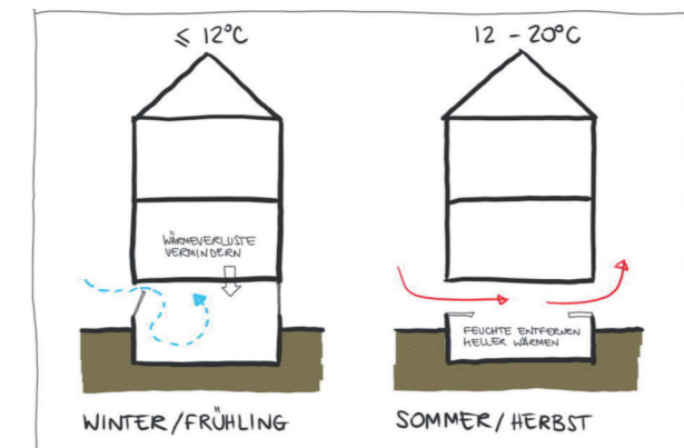
Abb. 8. Lüftungsstrategie Untergeschosse
