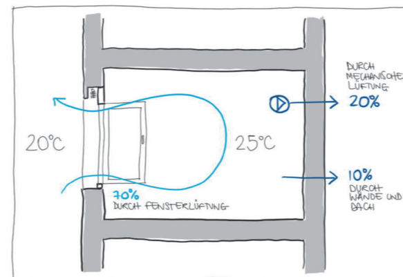
Abb. 6. Wärmeabfuhr aus dem Raum
